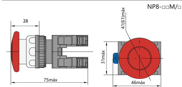
Dimensiones (mm)
