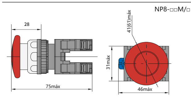
Dimensiones (mm)
