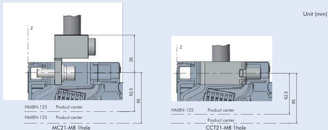
NM8N-125 Cable connector
