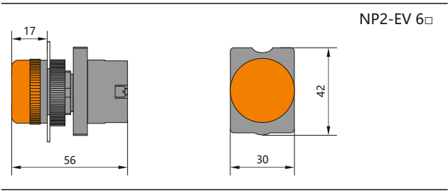
Dimensiones (mm)
