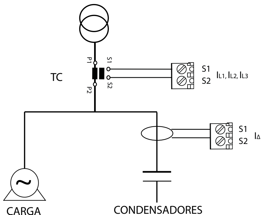
Figura 9: Conexión del transformador de corriente de fugas ( I_{\Delta} ).
