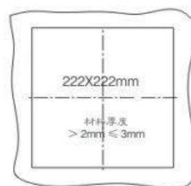
mounting dimension 安裝開口尺寸圖
