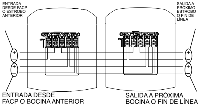
FIGURA 2. CABLEADO DE PRODUCTOS DE 4 CABLES:
